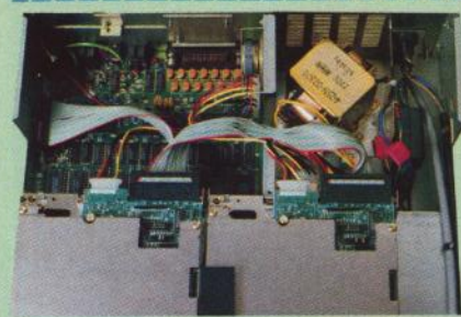
Sur la MBC 555 de Sanyo, on ne peut ajouter de cartes d'extension. ▼
